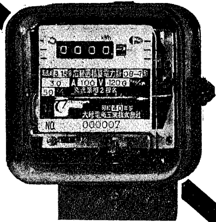
OB-7型広範囲单相積算電力計
